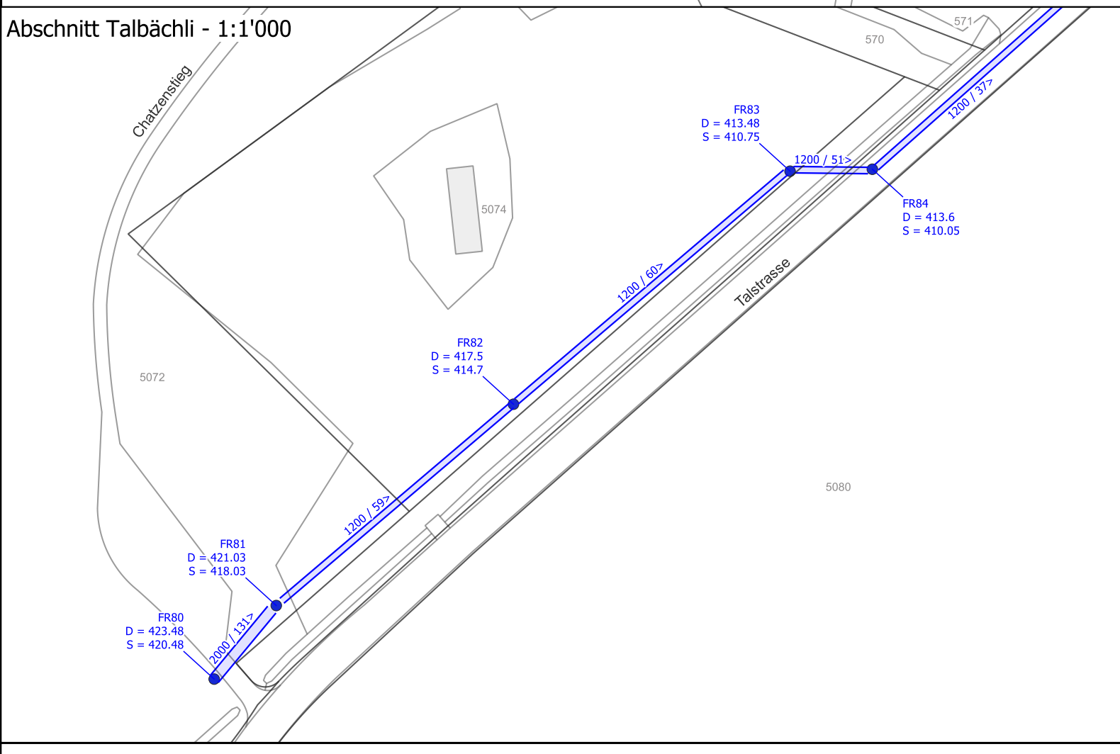
Abschnitt Talbächli - 1:1'000
